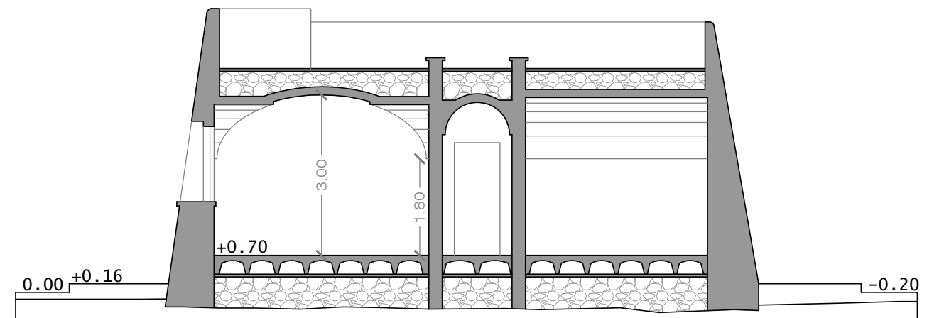
sezione b.b.
