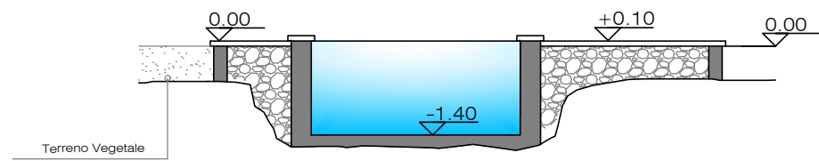
SEZIONE A B Scala 1:100
