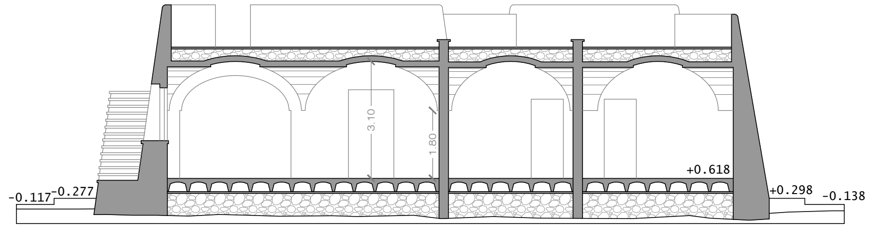
sezione a.a.
