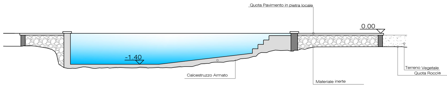
SEZIONE C D Scala 1:100
