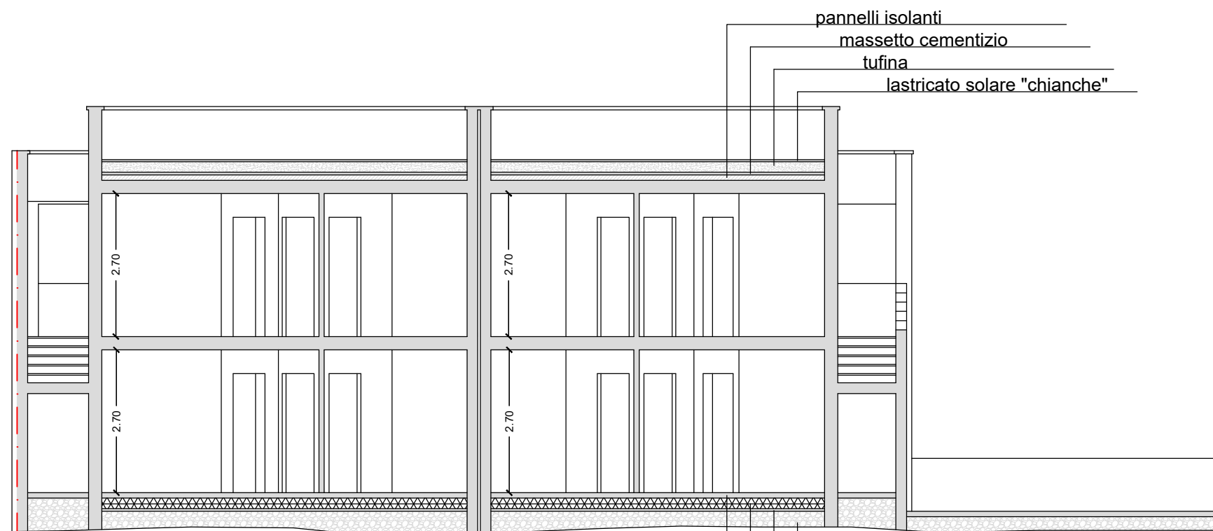
sezione a.b.
