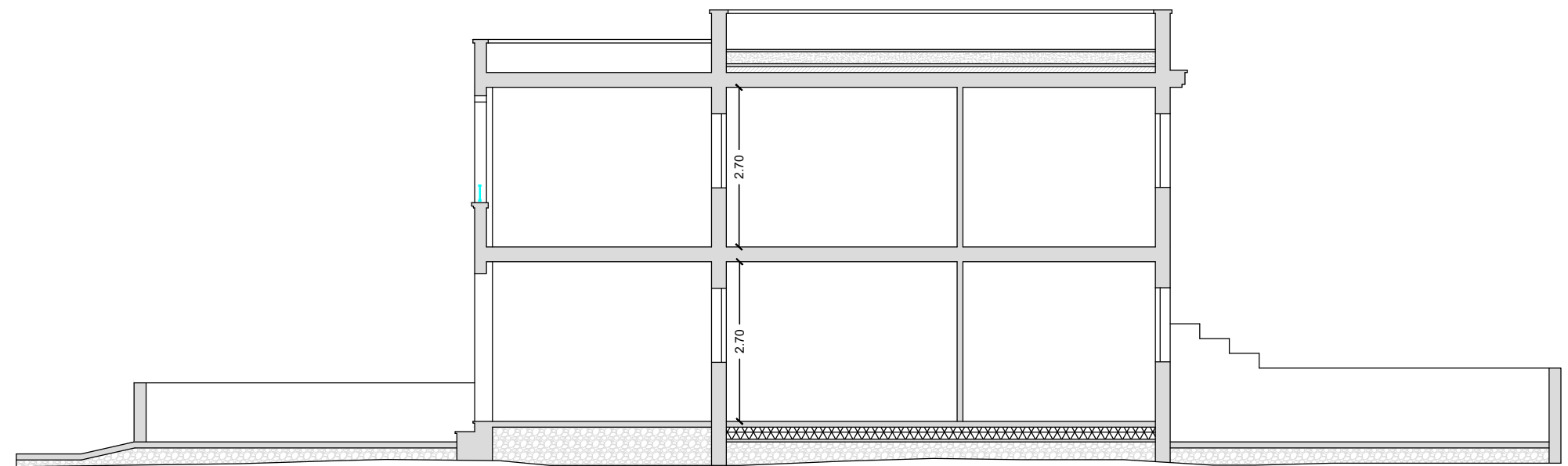
sezione c.d.
